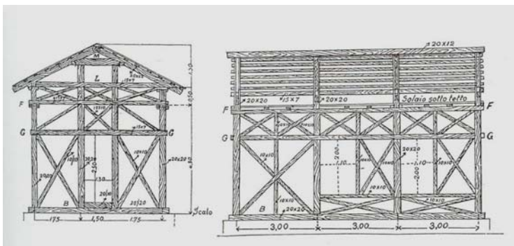
Un tipico schema costruttivo delle intelaiature di legno da inserire nelle "case baraccate" secondo i disegni dell'architetto Vincenzo Ferraresi, pubblicato nella "Historia de' tremuoti ..." di Giovanni Vivenzio, Stamperia Regale, Napoli, 1873 (dal volume di Clementina Barucci, La Casa Antisismica ).
